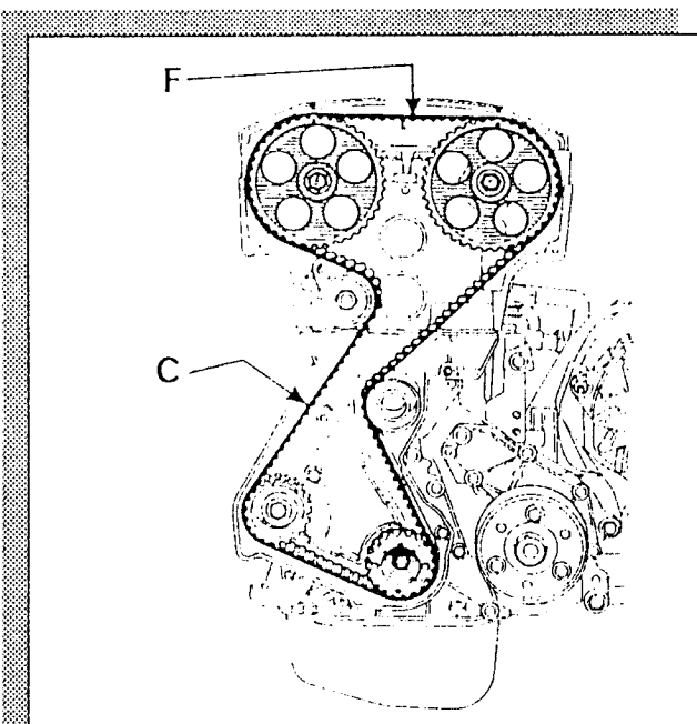
Contrôle tension courroie
