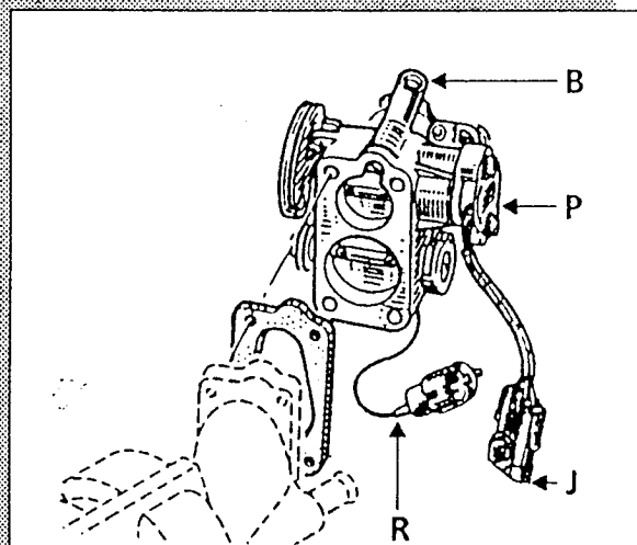
Boîtier papillons
