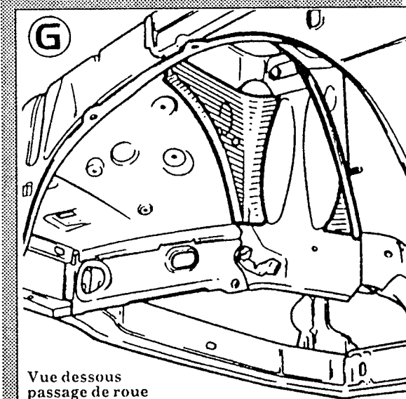
RENFORTS CHAPELLE
