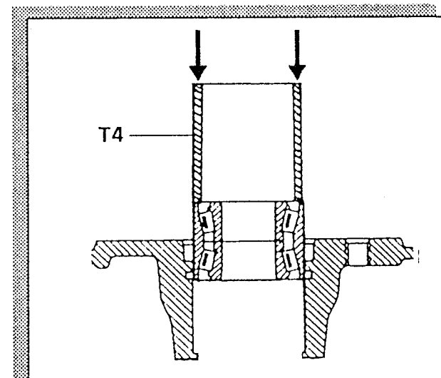
Repose roulement arrière
