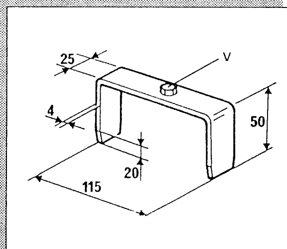
Outil de dépose - Pompe ess.
