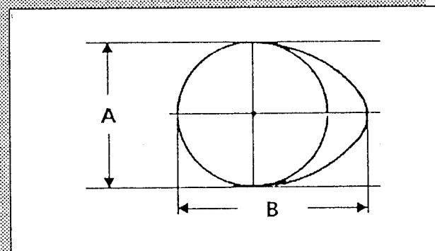
Cotes contrôle cames
