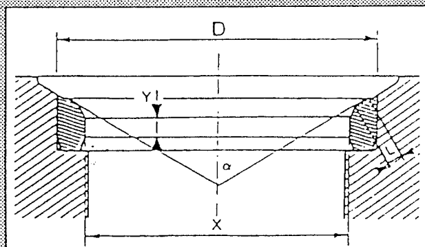
Cotes de contrôle des sièges de soupapes
