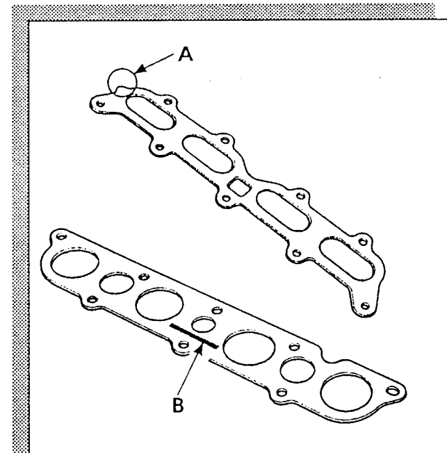
Indexage joints collecteurs
