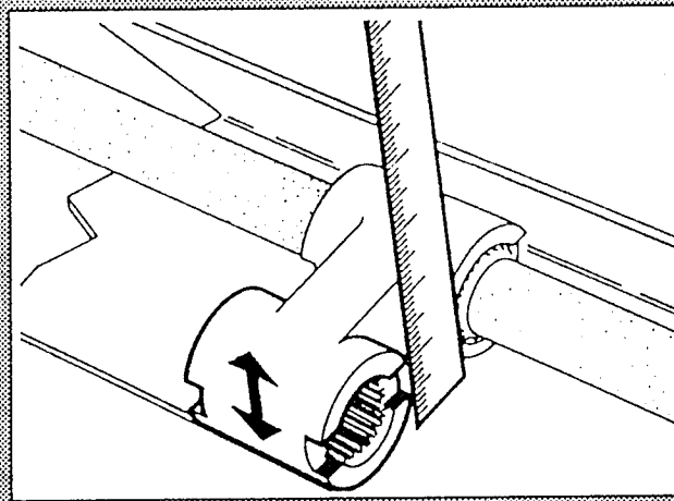
Mesure jeu de jumelle
