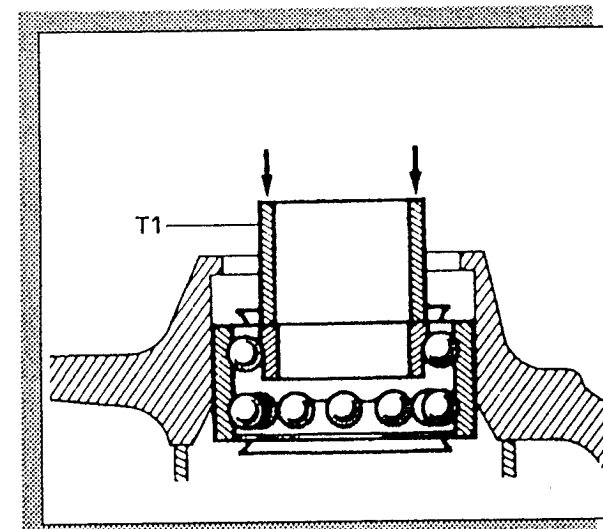
Dépose du roulement
