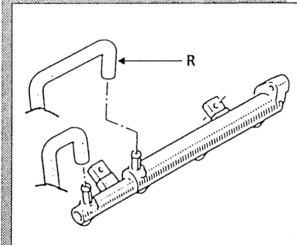
Alimentation rampe
