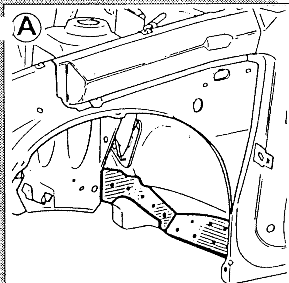
RENFORTS LONGERON TRAVERSE LATERALE AVANT
