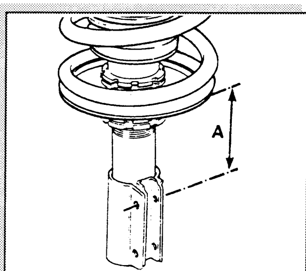
Préréglage amortisseur
