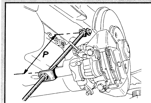
Préréglage train arrière
