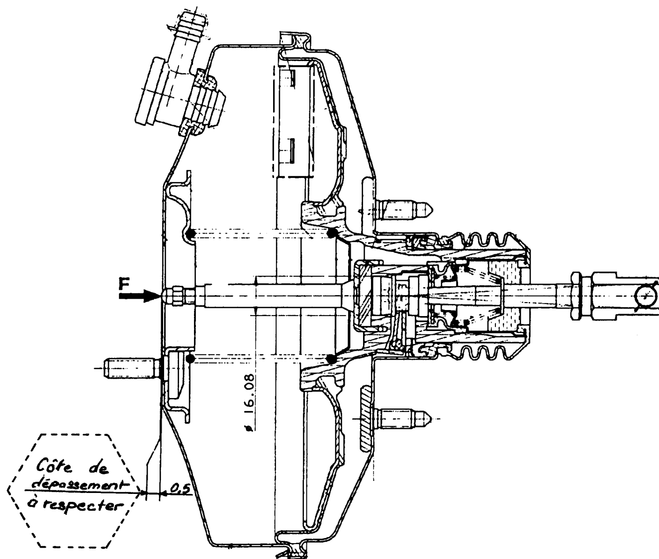
Réglage Master-Vac
