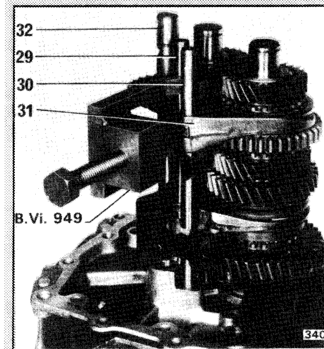
Montage fourchette 3/4
