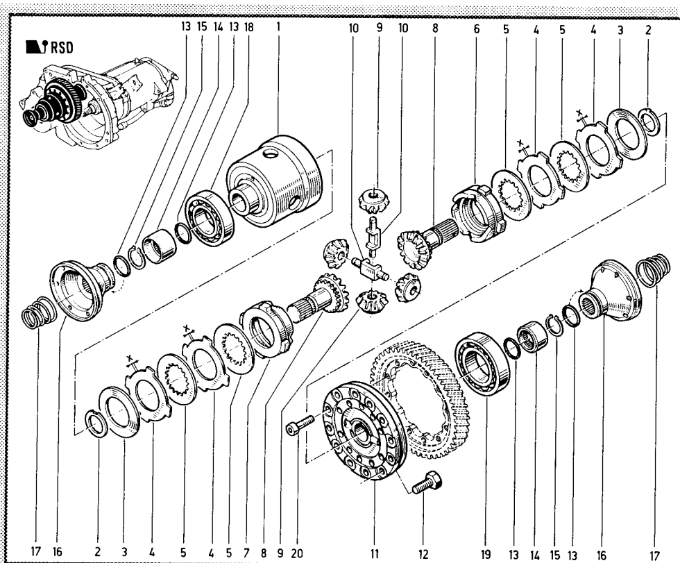
Ensemble différentiel
