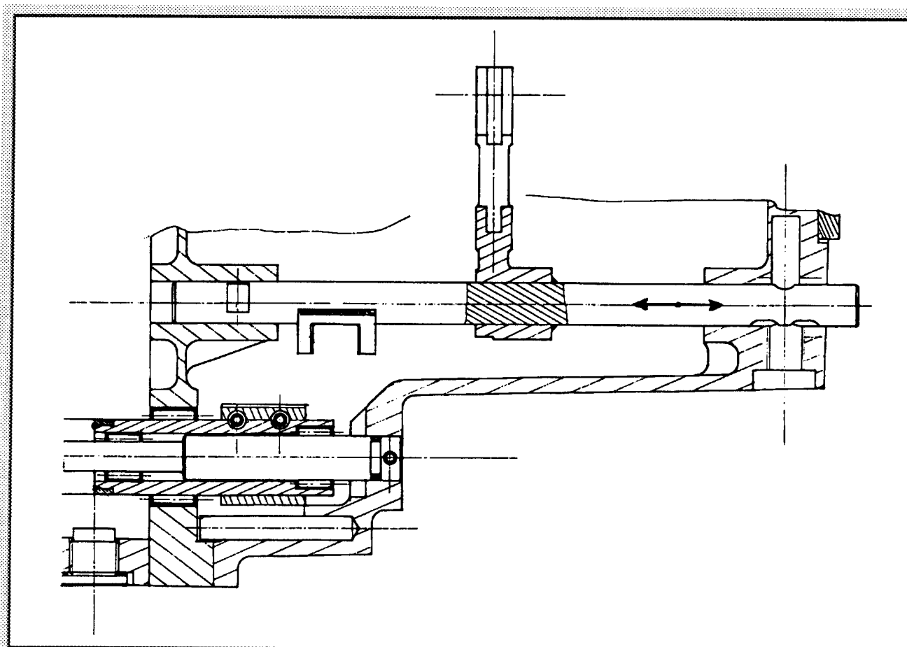
Montage fourchette 1/2
