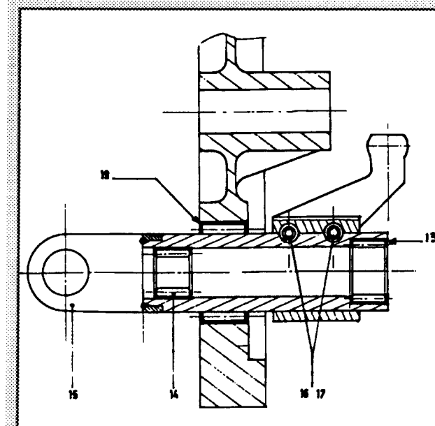
Montage sélecteur de vitesse
