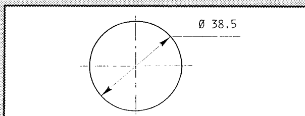
Conduit d'échappement
