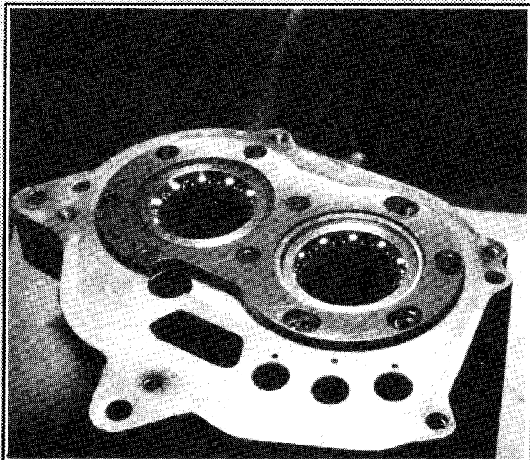
Plaque d'appui roulements
