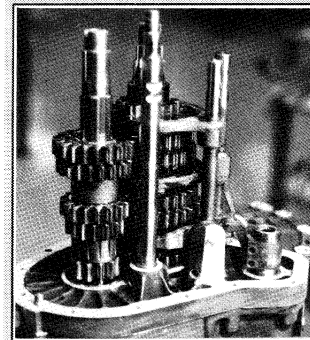
Montage pignonnerie
