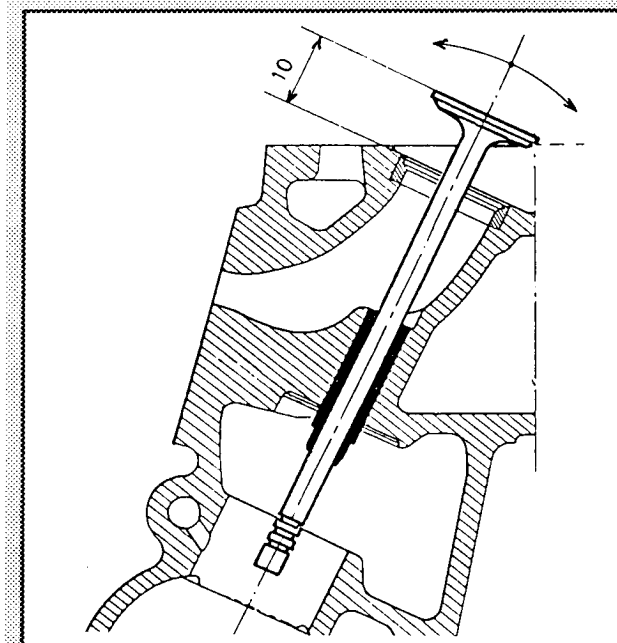
Contrôle jeu de basculement
