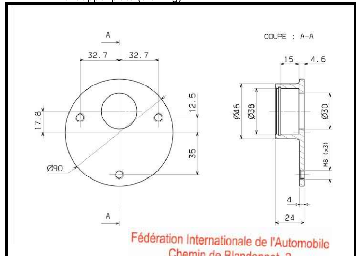
Tolérances : +/- 1 mm
