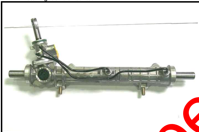
CD1) Crémaillère de direction démontée Steering rack dismounted
